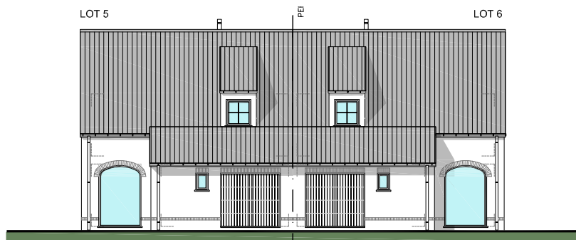
VOORGEVEL
