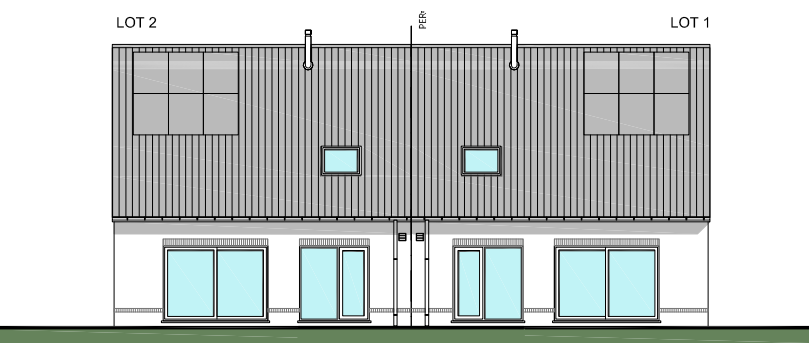
ACHTERGEVEL
