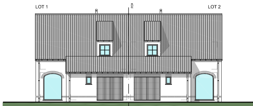
VOORGEVEL
