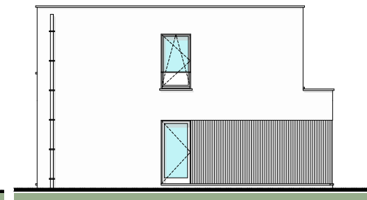
ZIJGEVEL LINKS
