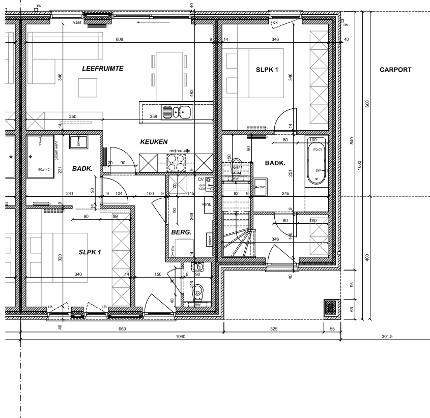
GELIJKVLOERS HOOFDWONEN: OPP. 33,60 M 2 ZORGWONEN: OPP. 63,52 M 2 CARPORT: OPP. 21,10 M 2
