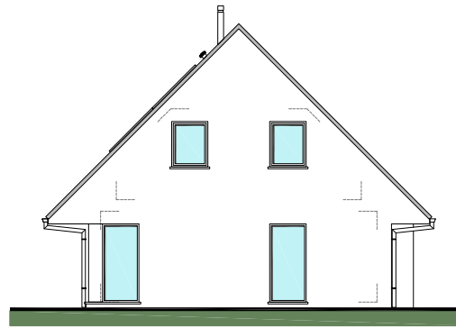
ZIJGEVEL LINKS
