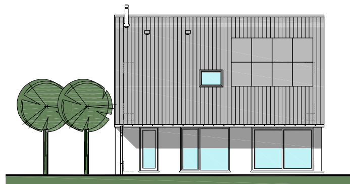
ACHTERGEVEL
