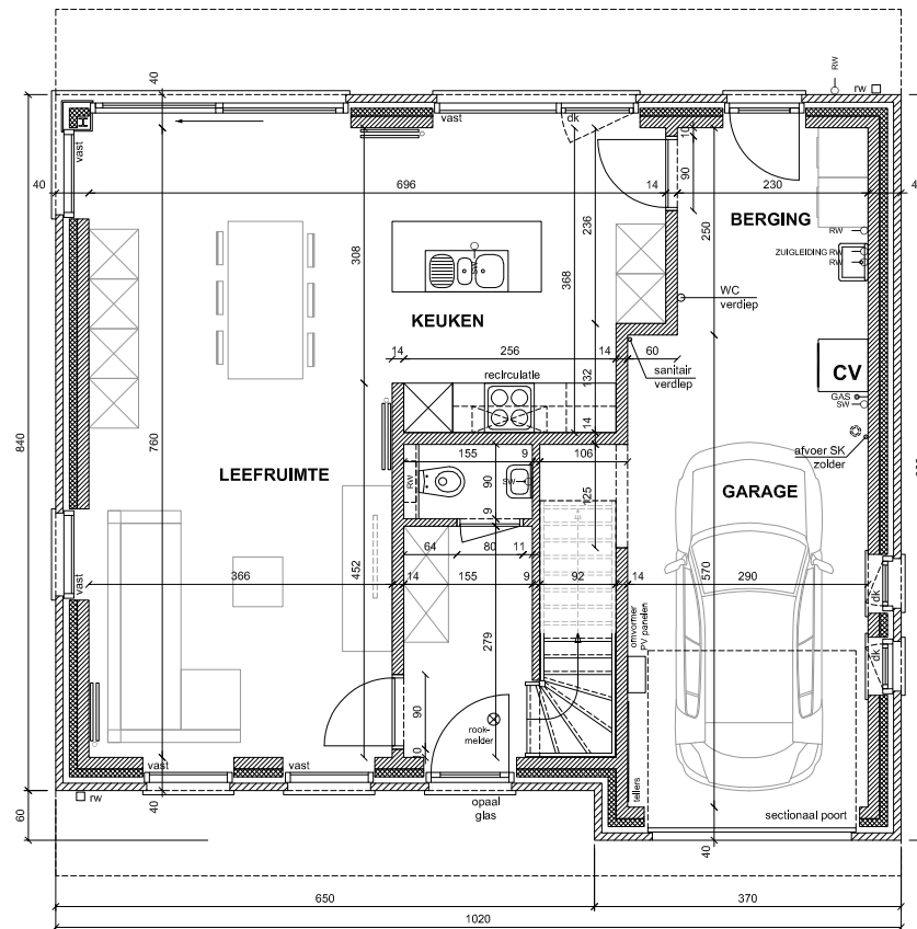
GELIJKVLOERS OPP. 87.9 M 2
